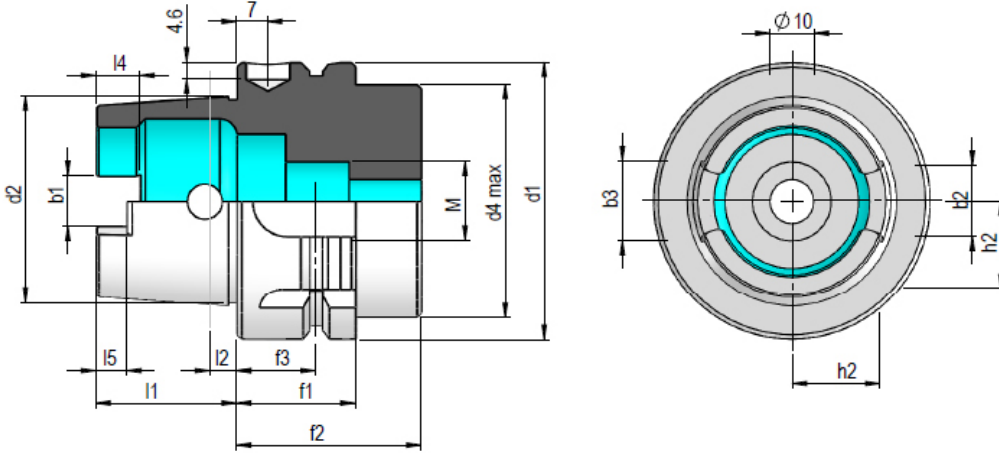
Kegel 1:10
